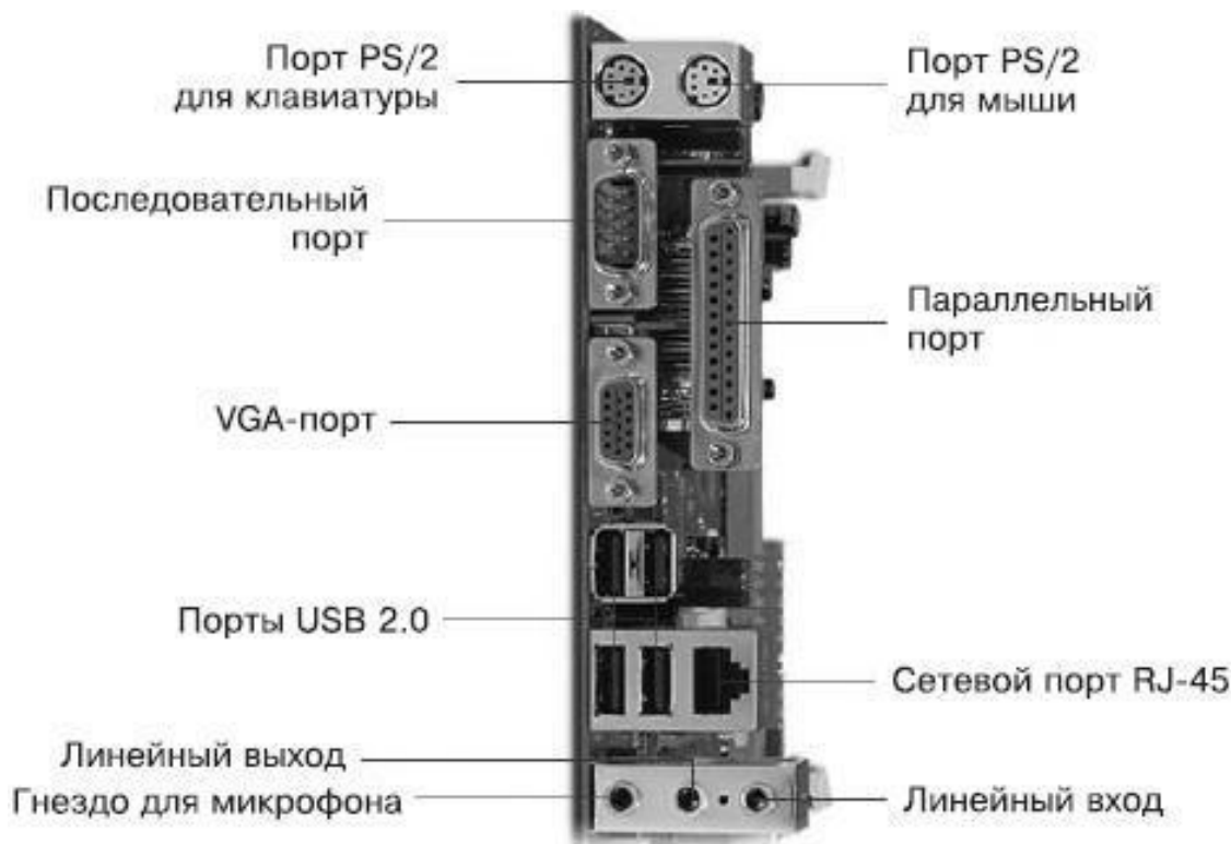
Рис. 0.4. Разъемы на задней стороне компьютера
