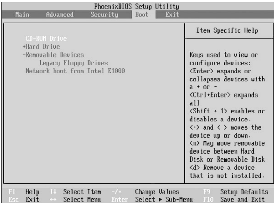
Рис. 2.1. Изменяем порядок загрузки с устройств
