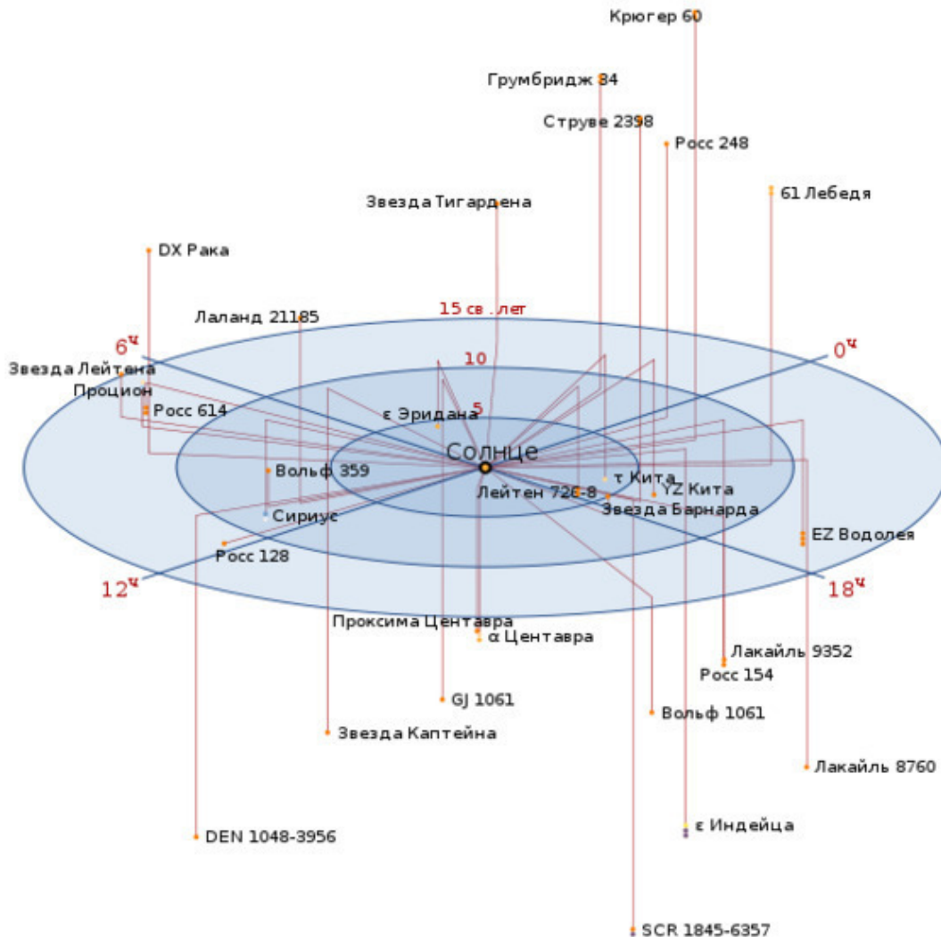
Схема расположения ближайших звезд
