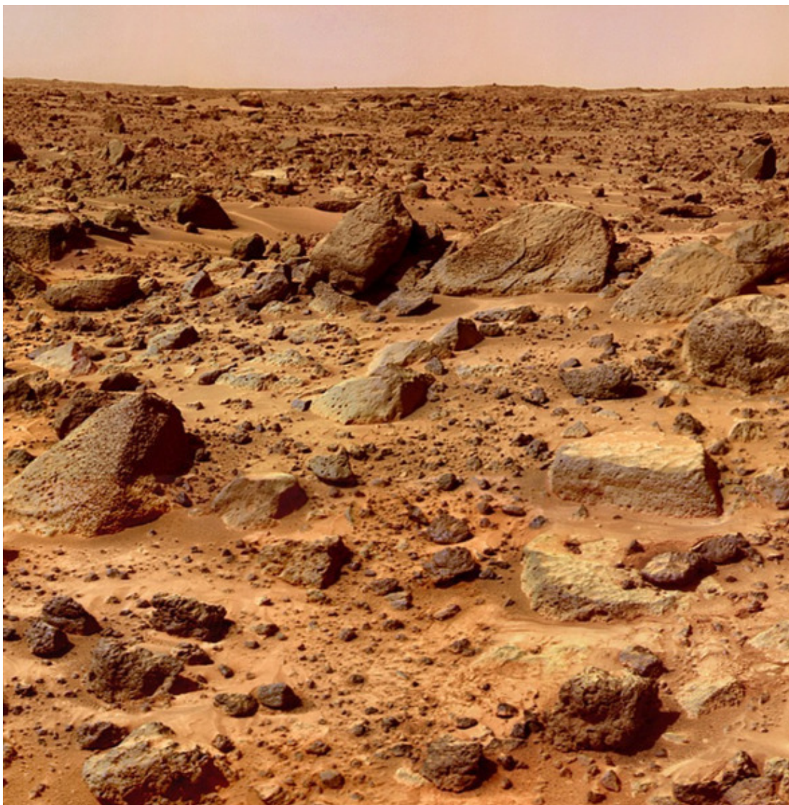
Марсианский пейзаж
