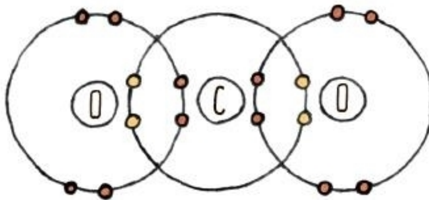
молекула углекислого газа
