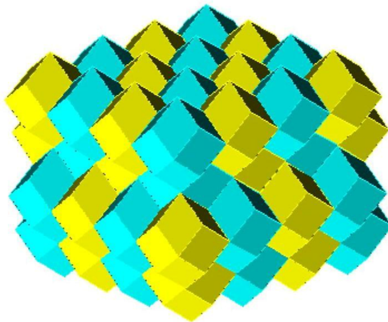
Рисунок 8. Четырехслойный фрагмент пространства
