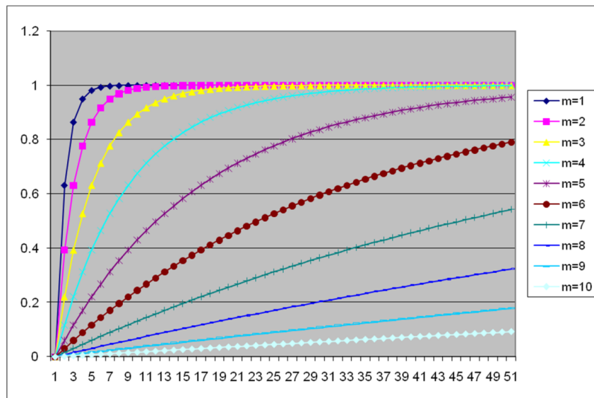
Рисунок 11. Зависимость плотности эфира – \rho t от расстояния до центра объекта – t для разных значений его массы – m
