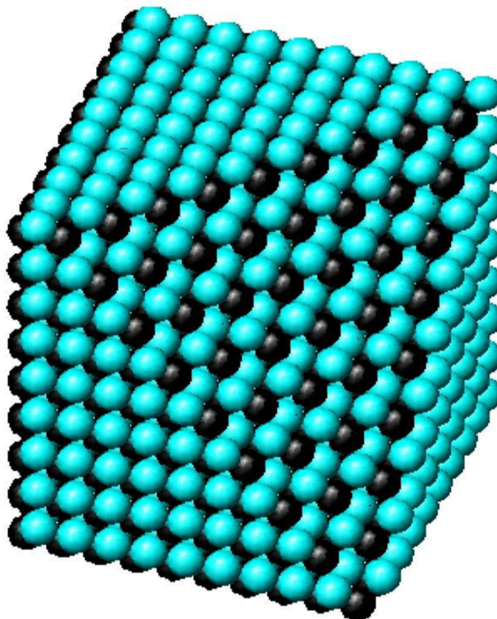
Рисунок 1. Пространство, заполненное шарами
