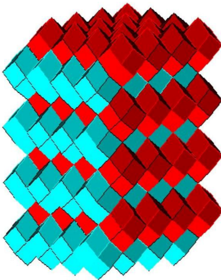
Рисунок 3. Квантованное пространство
