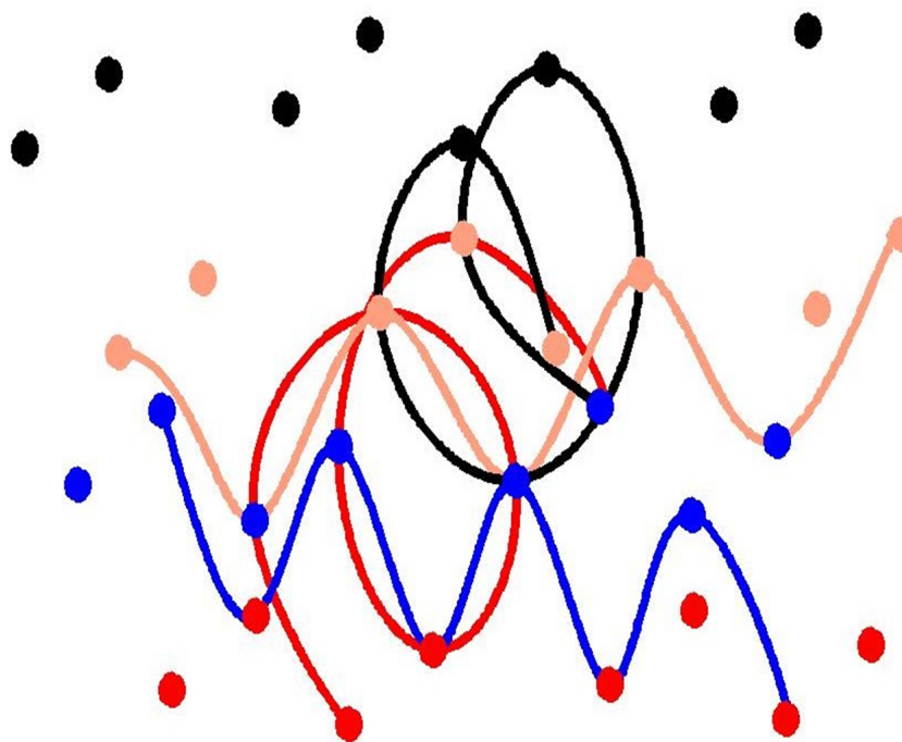
Рисунок 10. Возможные траектории движения точки в пространственной сети
