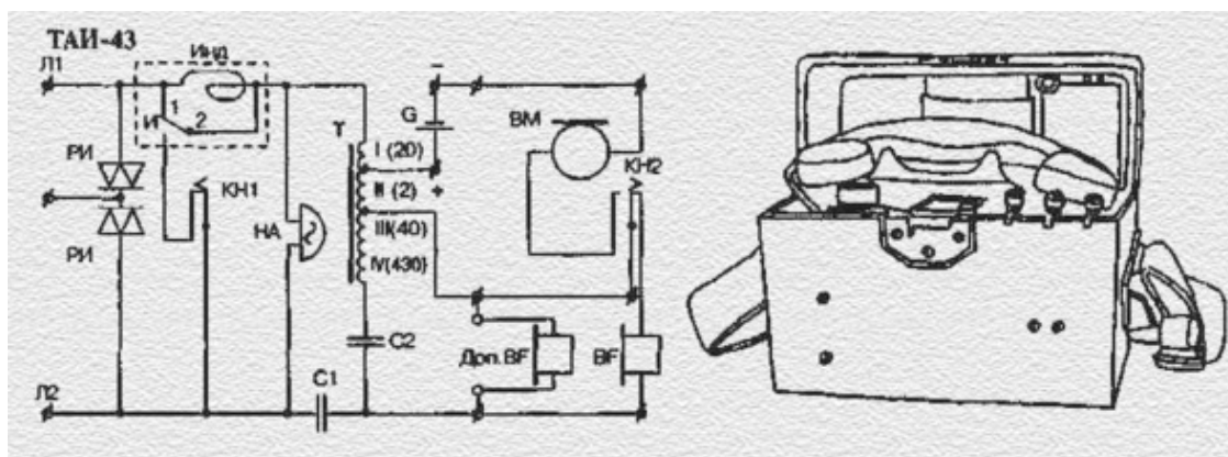
Телефонный аппарат ТА 43 (образца 1943г.)
