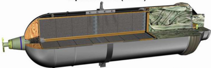
Осветительная авиационная бомба САБ-100-55 индекс 13-С-55 чертеж 05941М (1941г.)
