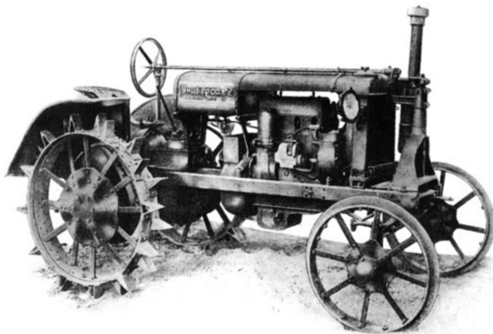
Трактор «Универсал-2»
