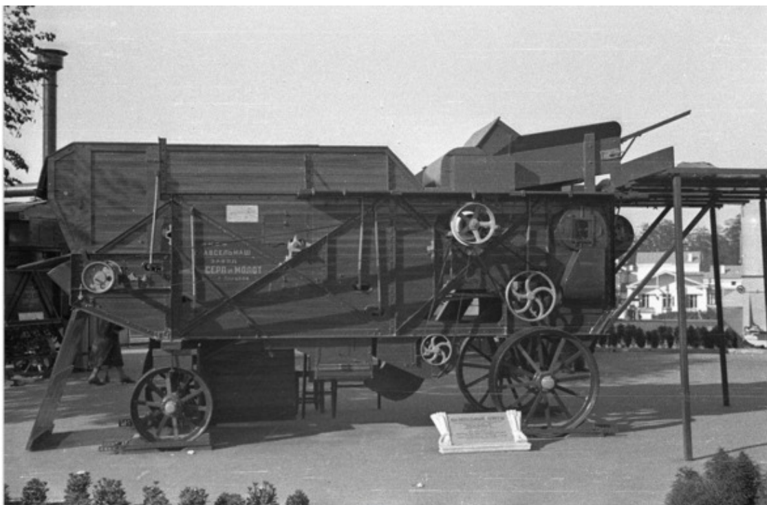
Молотилка МК-100
