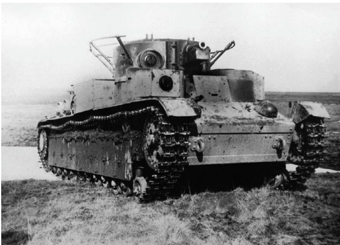
Общие виды танка Т-28 выпуска 1936 года. Машина имеет колпак над вентилятором с жалюзи и одностворчатым люком, шаровую установку в нише башни, два люка в крыше башни и измененную (по сравнению с танками предыдущих серий) укладку ЗИП.
