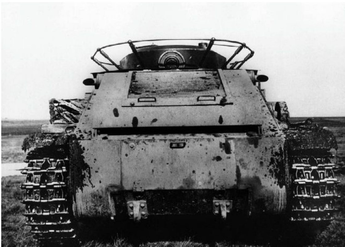
Танк Т-28 выпуска 1936 года, вид сзади. Хорошо виден колпак над вентилятором с жалюзи и одностворчатый люк, шаровая установка в нише башни.
