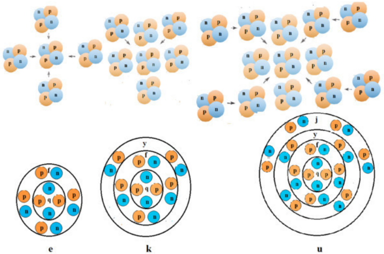
Рис. 2. Схема образования ядер неона, кремния и железа. е – неон, к – кремний, u – железо
