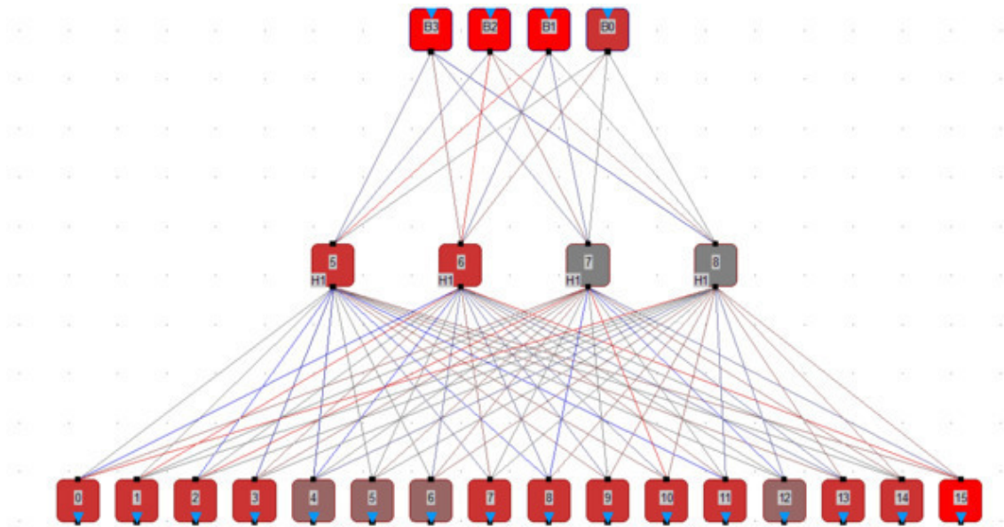
Рис.2 Нейросеть из файла «Decoder4To16.mbn»
