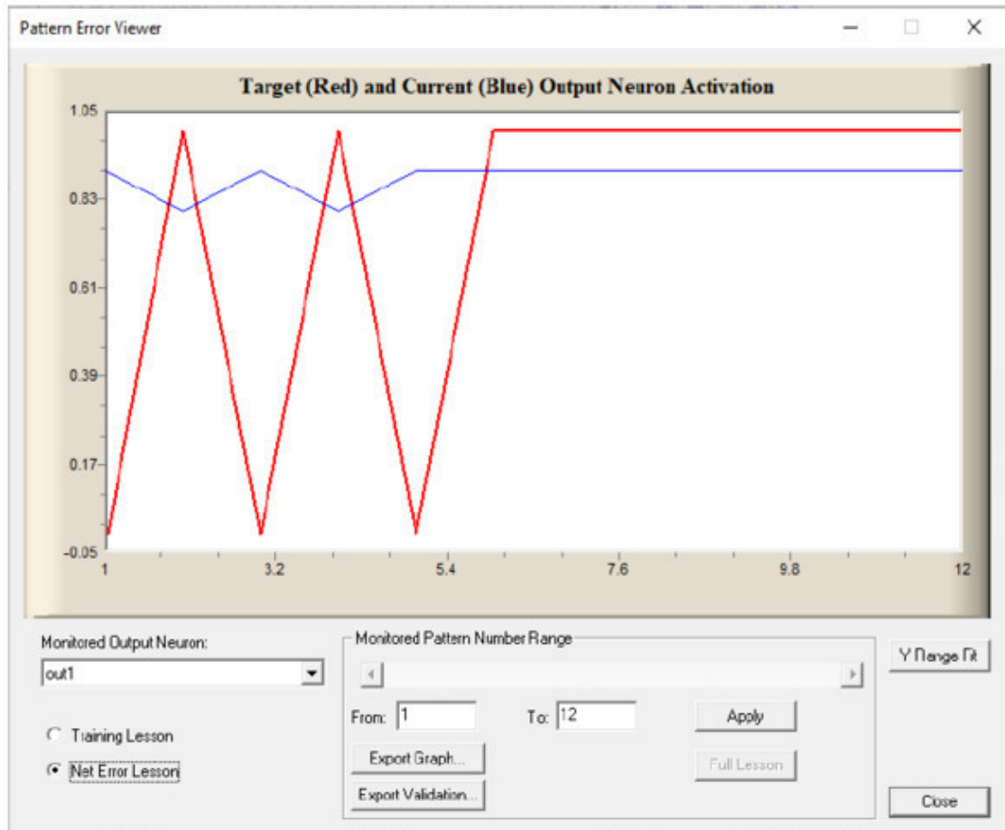
Рис.31 Процесс обучения нейросети
