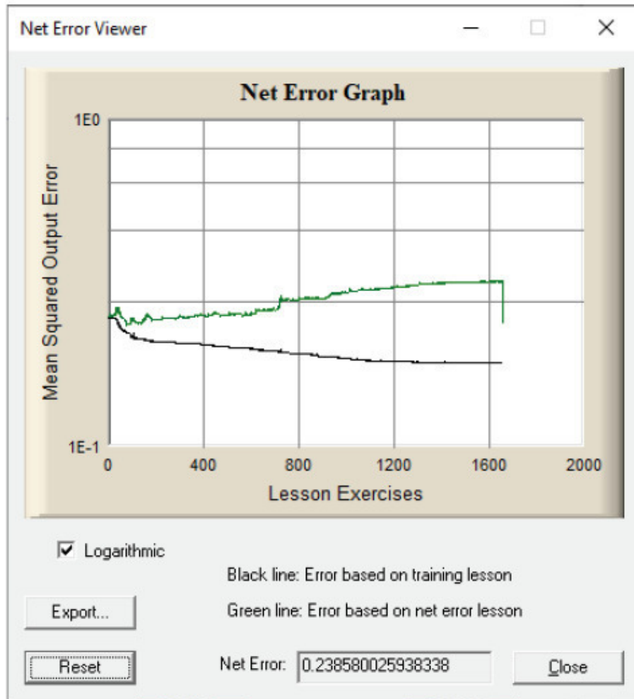
Рис.30 Ход обучения преобразователя кодов
