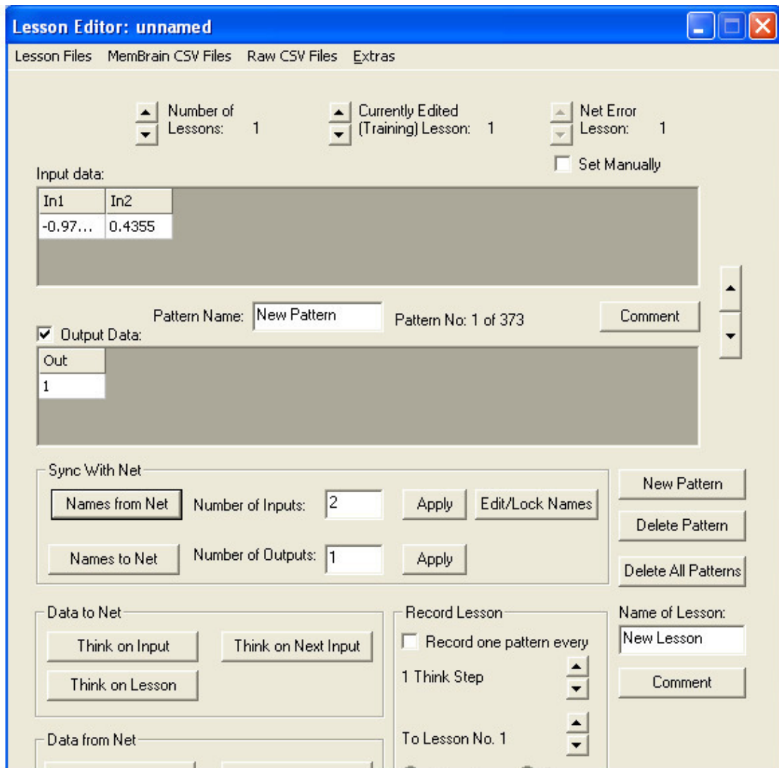
Рис.14 Загружен обучающий файл
