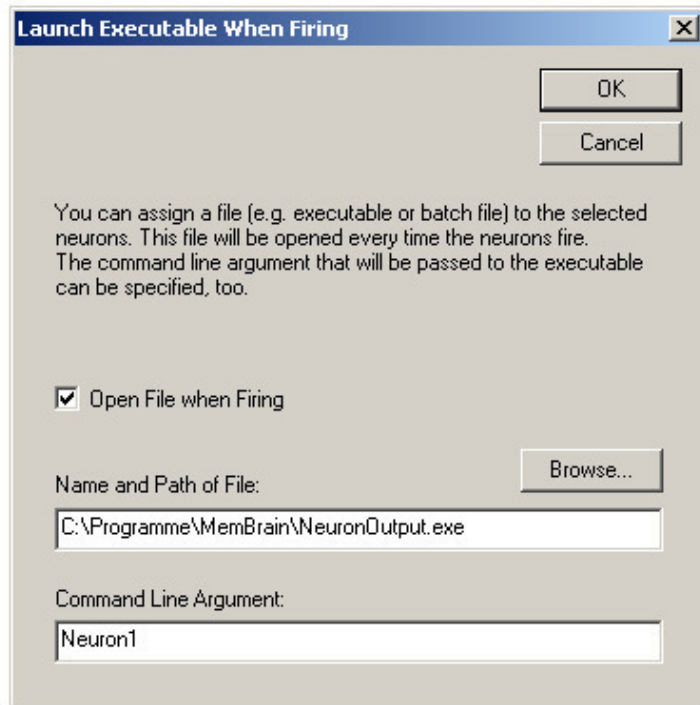
Рис.25 Настройка зажигаемого файла
