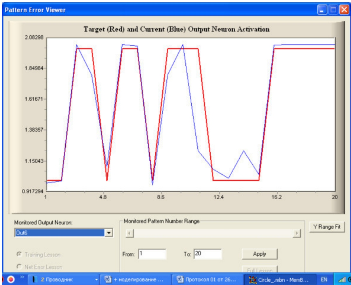
Рис.18 Ход обучения нейросети
