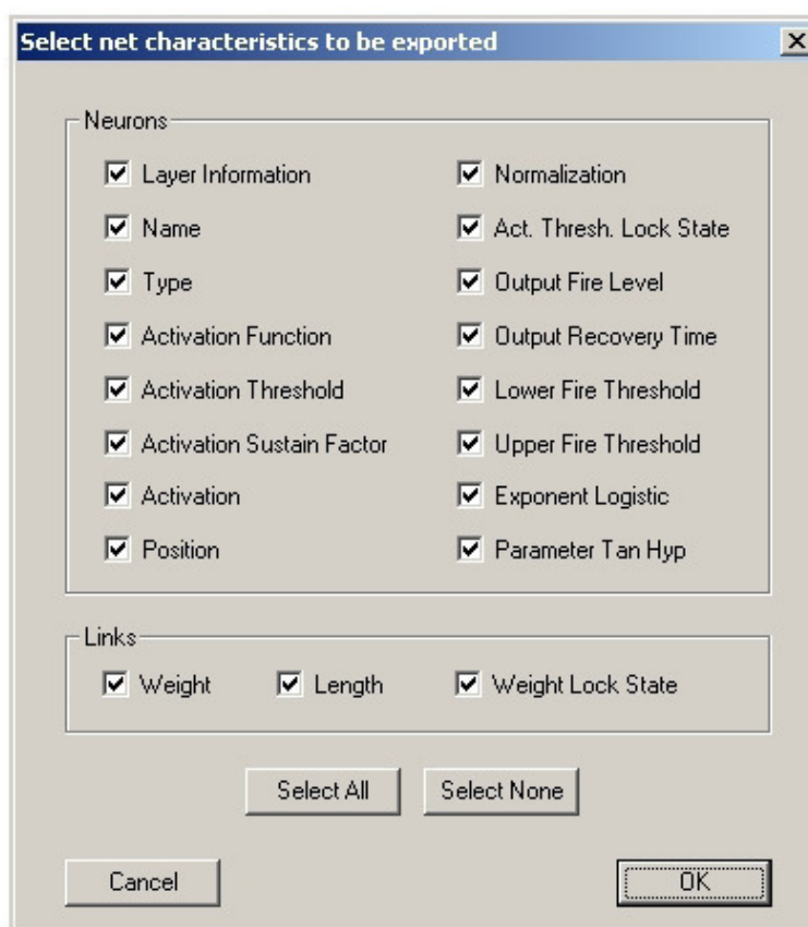
Рис.12 Настройка экспорта нейросети
