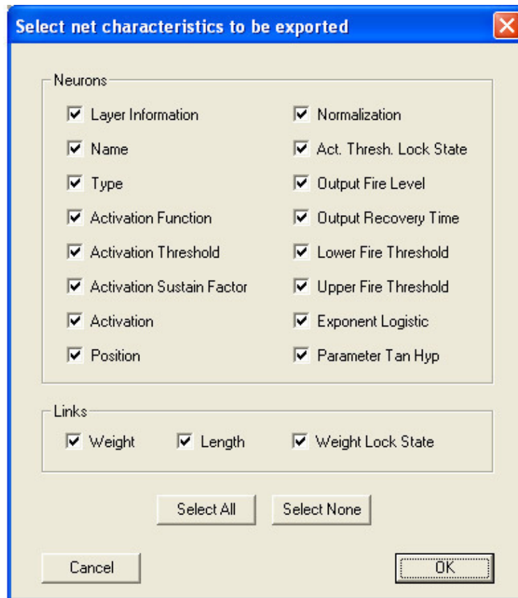
Рис.19 Подготовка экспорта обученной нейросети
