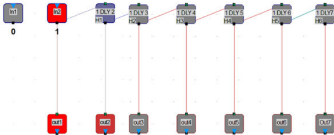
Рис.27 Схема преобразователя последовательного кода в параллельный
