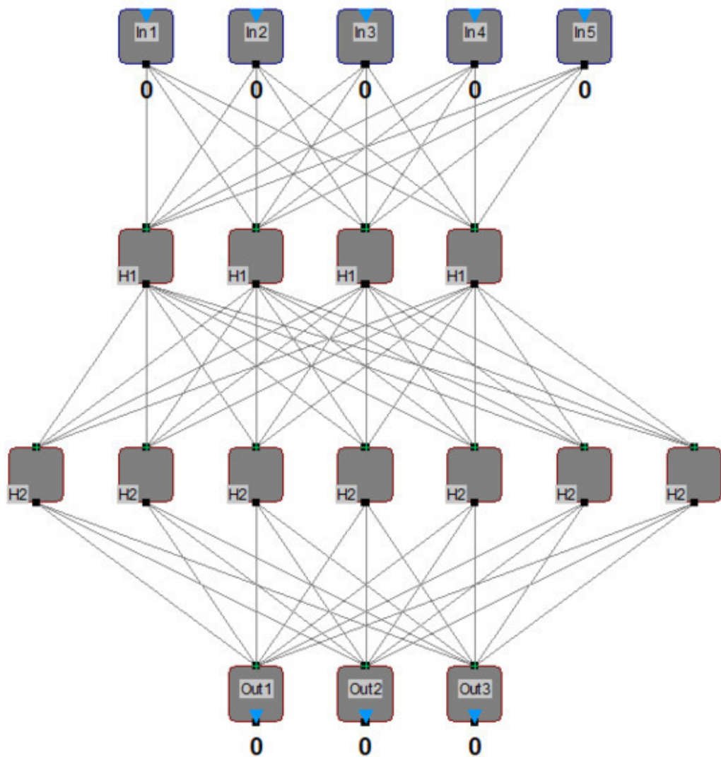
Рис.57 Схема созданной нейросети
