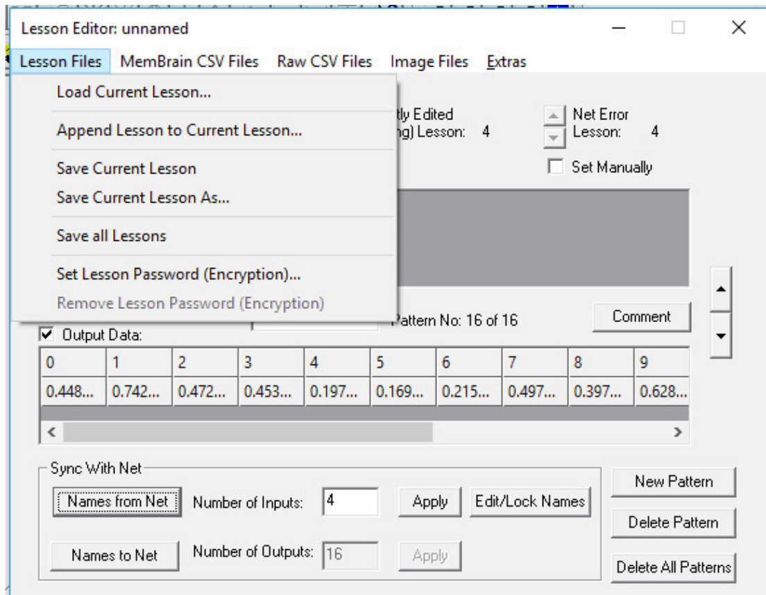
Рис.11 Загрузка mbl-файла
