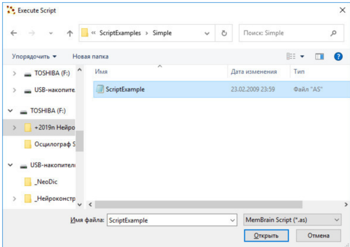
Рис.9 Имя скрипта
