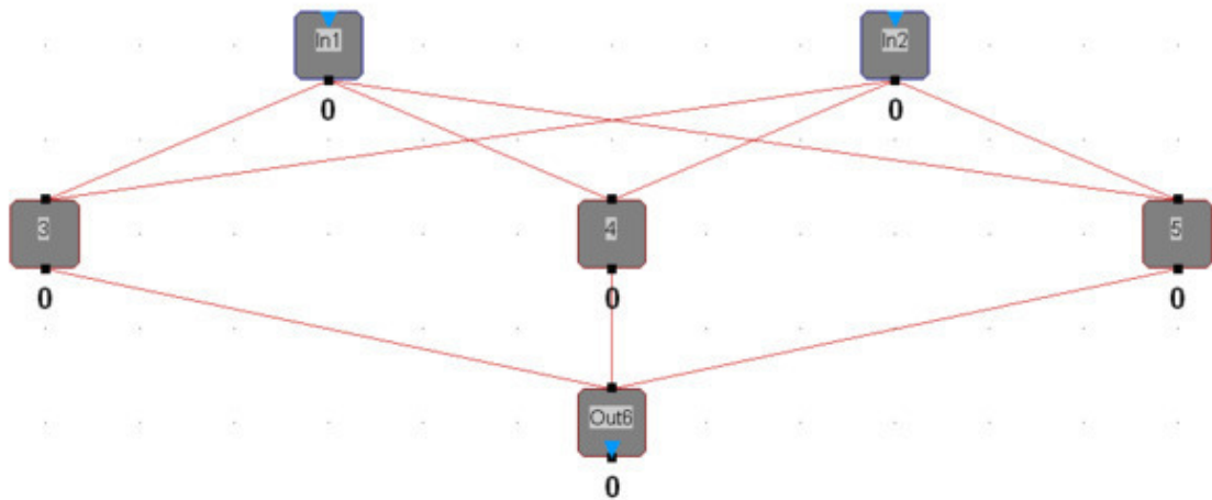
Рис.13 Нейросеть загружена
