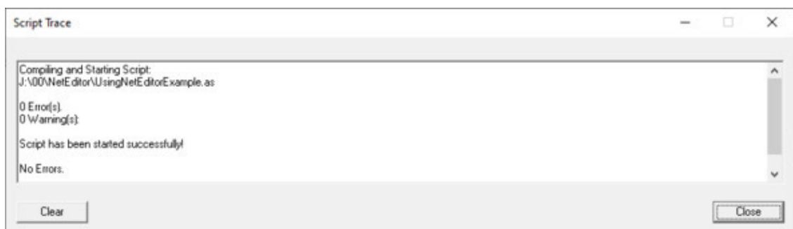
Рис.55 Трасса скрипта
