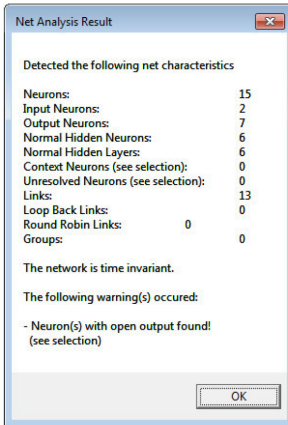
Рис.28 Характеристики нейросети
