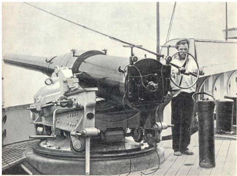
6-ти-дюймовая дальневойная пушка въ 35 калибровъ на крейсере.
