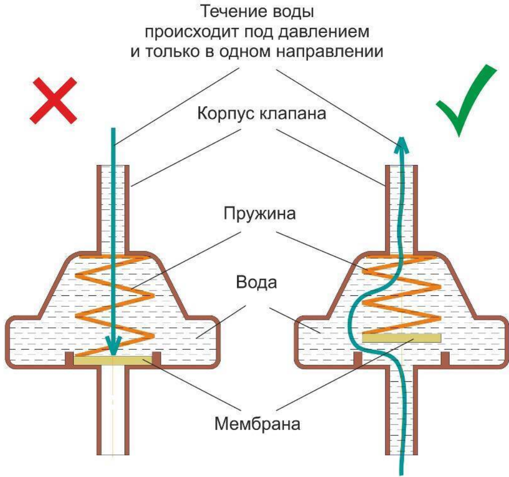
Устройство клапана
