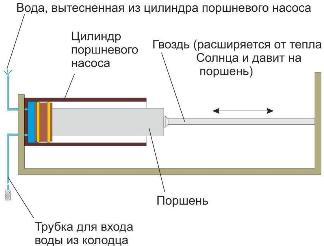
Схема поршневого насоса, работающего от Солнца, с использованием гвоздя
