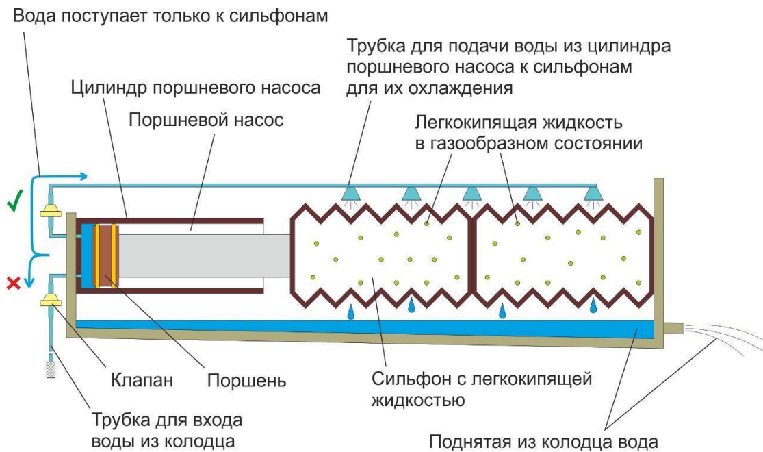
Схема поршневого насоса, работающего от Солнца (сифоны разжаты)
