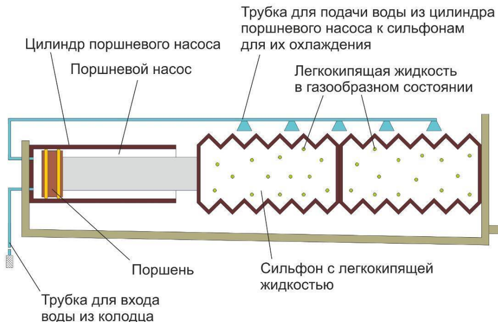
Схема поршневого насоса, работающего от Солнца (сифоны разжаты)
