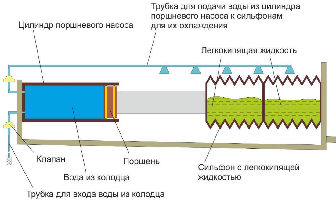
Схема поршневого насоса, работающего от Солнца (сифоны сжаты)
