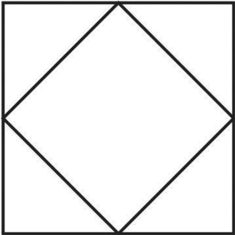
Квадрат, вписанный в квадрат
