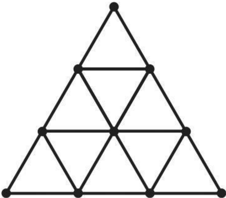
Сакральный треугольник с десятью точками
