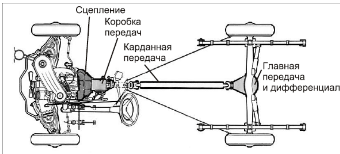
Рис. 1.1. Классическая схема размещения агрегатов и узлов автомобиля
