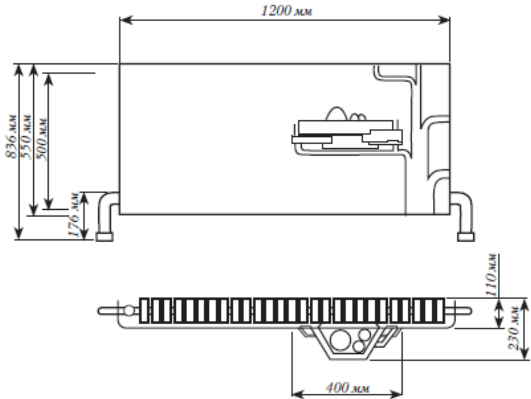
Рис. 14. Размеры украшения для батареи
