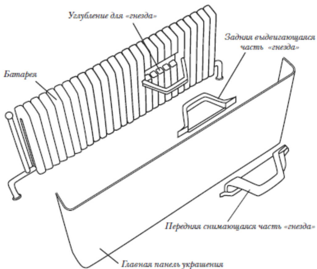
Рис. 13. Конструктивное устройство украшения, для батареи
