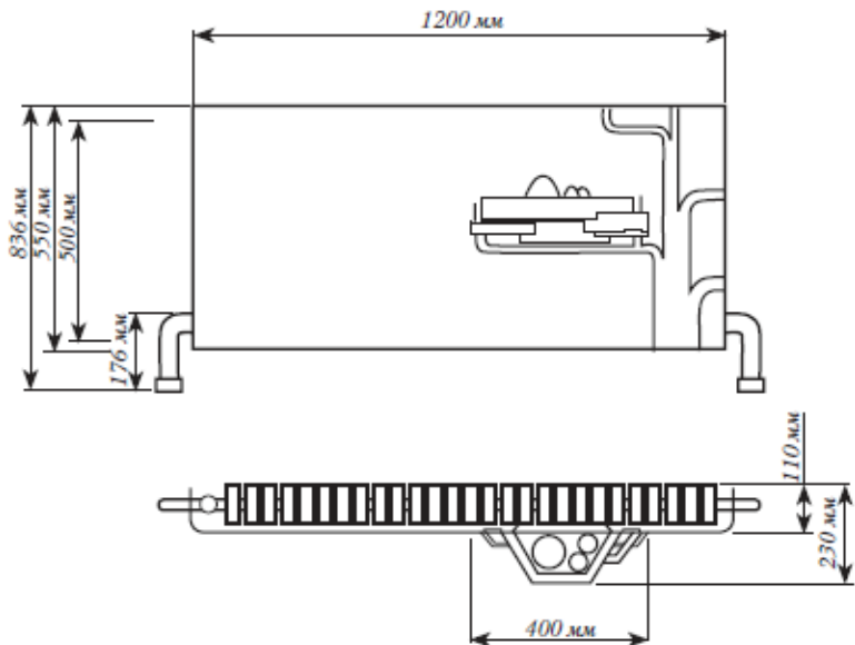
Рис. 14. Размеры украшения для батареи
