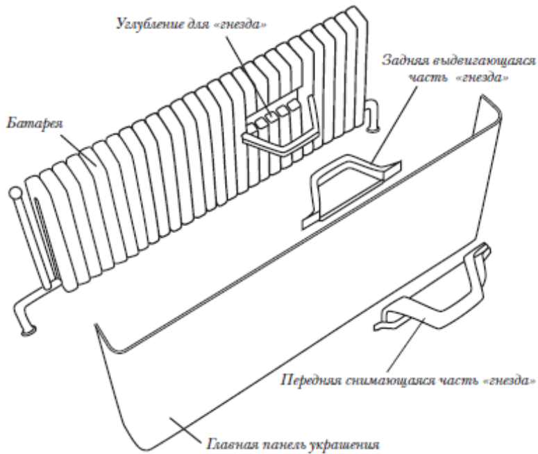
Рис. 13. Конструктивное устройство украшения, для батареи
