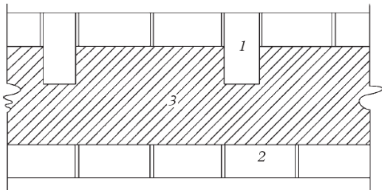
Рисунок 2. Модифицированная колодцевая кладка: 1 – наружная верста; 2 – внутренняя верста; 3 – утеплитель
