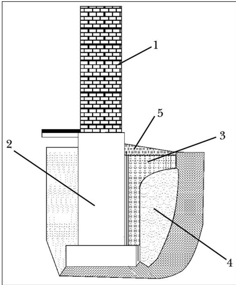
Рисунок 6. Утепление фундамента: 1 – стена; 2 – фундамент; 3 —утеплитель; 4 – песок; 5 – отмостка
