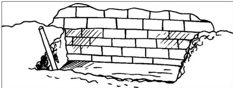
Рисунок 4. Шурф для исследования фундамента
