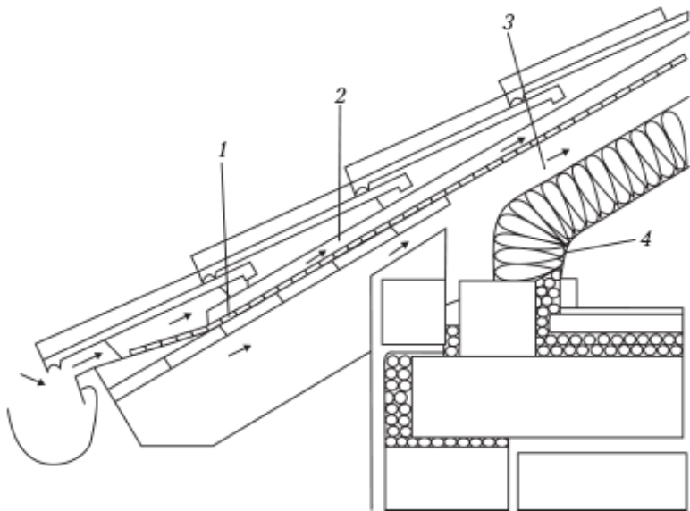
Рис. 63. Общая схема утепленной крыши: 1 – подкровельная гидроизоляция; 2 – контробрешетка; 3 – теплоизоляция; 4 – паронепроницаемый слой
