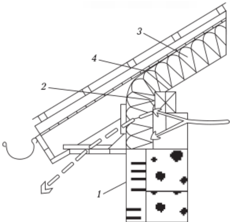
Рис. 64. Изоляция примыкания коленчатой стенки к крыше: 1 – утеплитель стены; 2 – мауэрлат; 3 – утеплитель крыши (минвата); 4 – место, где нельзя обрывать утеплитель
