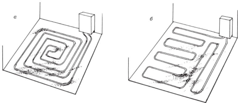
Рис. 55. Укладка труб: а) по спирали; б) змейкой
