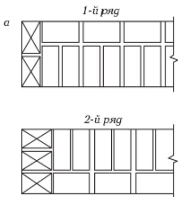
Рис. 29. Цепная кладка: а) кладка в полтора кирпича, б) кладка в два кирпича
