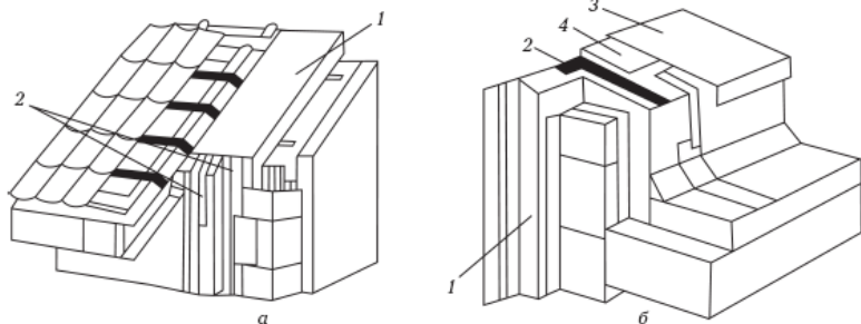
Рис. 67. Соединение с утеплителем стены утеплителя: а) скатной крыши; б) плоской крыши; 1 – утеплитель; 2 – армирующая сетка; 3 – жестяной фартук; 4 – уплотняющая лента из полиуретана
