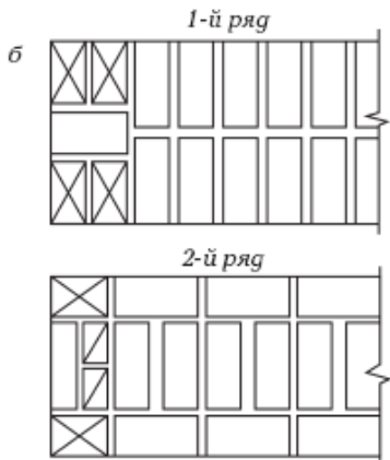
Рис. 29. Цепная кладка: а) кладка в полтора кирпича, б) кладка в два кирпича
