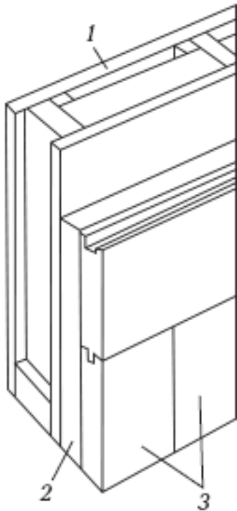
Рис. 49. Утепление щитовой стены: 1 – легкая стена из гипсоплит; 2 – утеплитель; 3 – гипсовая строительная плита
