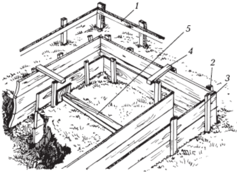
Рис. 28. Устройство деревянной опалубки: 1 – обноска; 2 – стойка; 3 – опалубка; 4 – перемычка; 5 – распорка
