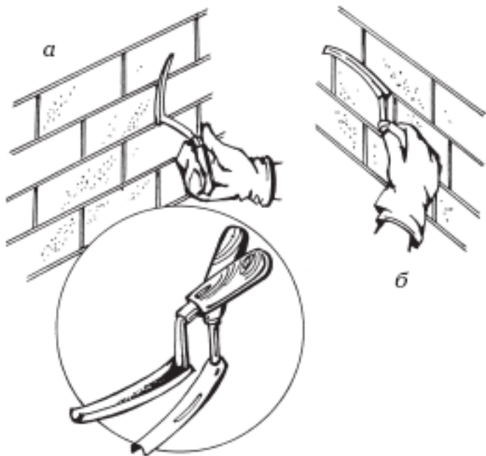
Рис. 31. Техника расшивки швов: а) вертикальных, б) горизонтальных
