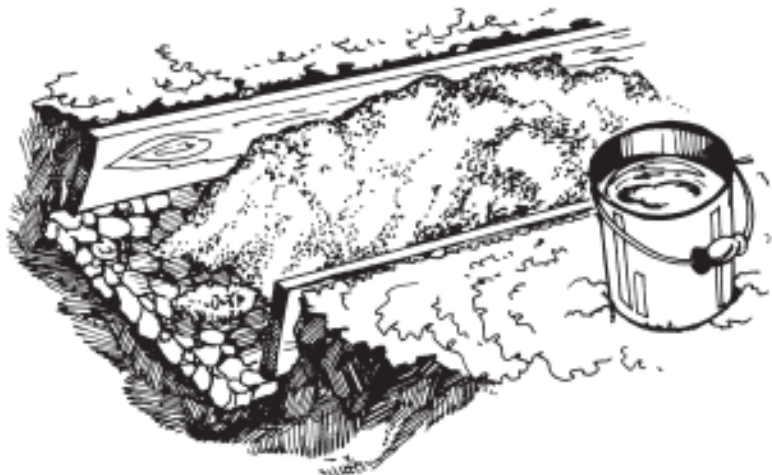
Рис. 14. Выравнивание основания
