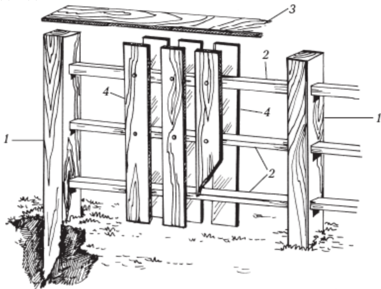
Рис. 24. Конструкция деревянного забора: 1 – брус для столбов 100 × 100 мм; 2 – брус 45 × 70 мм, 3 – доска 25 × 125 мм, 4 – крепление для прогонов (кронштейн или стальной уголок)
