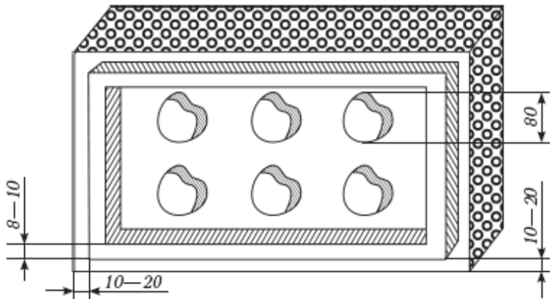
Рис. 39. Схема нанесения клеевого состава на утеплитель
