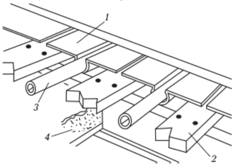
Рис. 57. Реечный тип монтажа водяного теплого пола: 1
