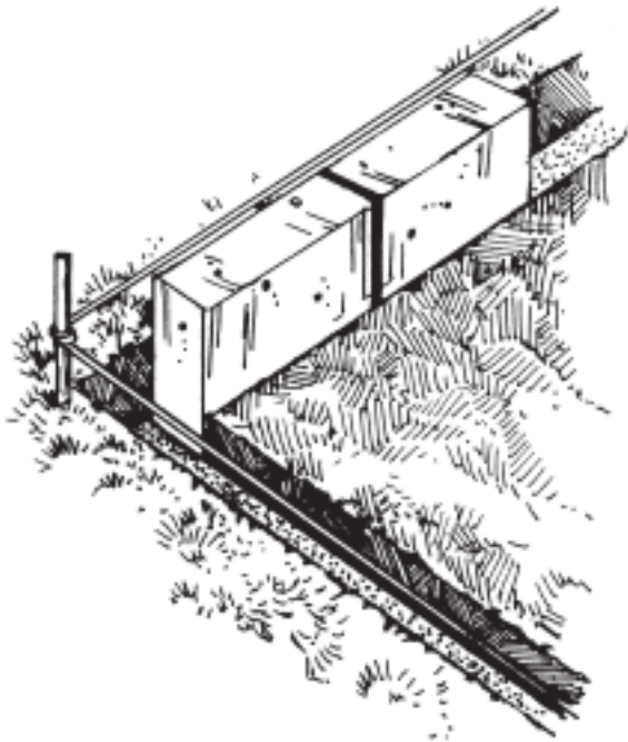
Рис. 20. Тип укладки на бетонной стяжке и песчаной подушке
