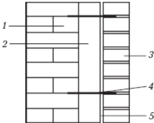
Рис. 33. Устройство слоистой кладки: 1 – несущая стена, 2 – теплоизоляция, 3 – облицовочный слой, 4 – закладные детали (связи), 5 – воздушный зазор
