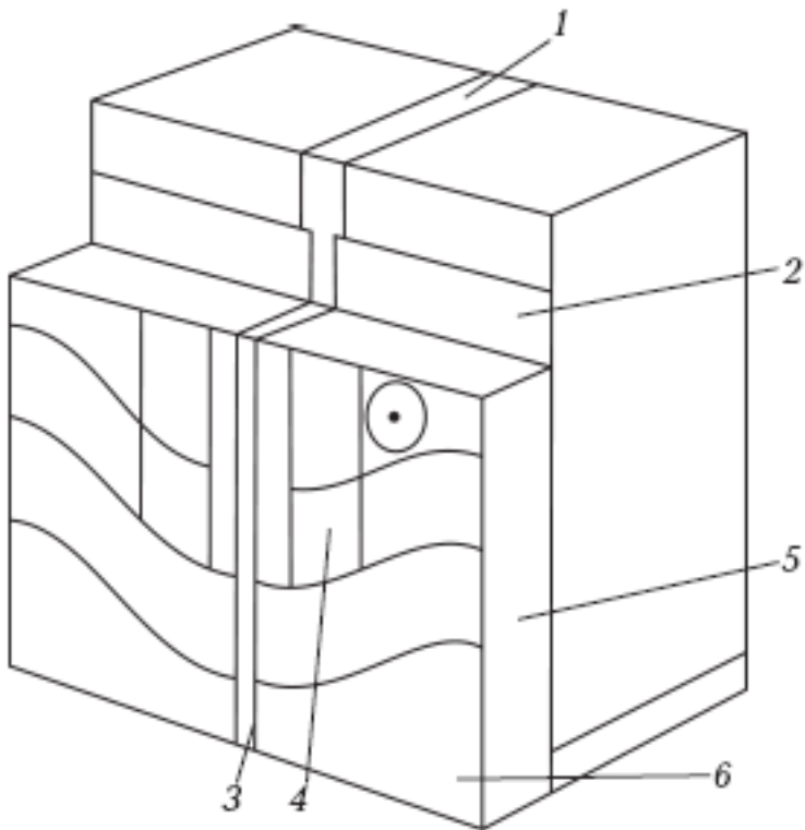
Рис. 44. Устройство деформационных швов: 1 – заполнение полоской минеральной ваты; 2 – клей; 3 – компенсационный шов, в котором размещены профиль и сетка; 4 – армирующая сетка, утопленная в клеевой раствор; 5 – утеплитель; 6 – штукатурка
