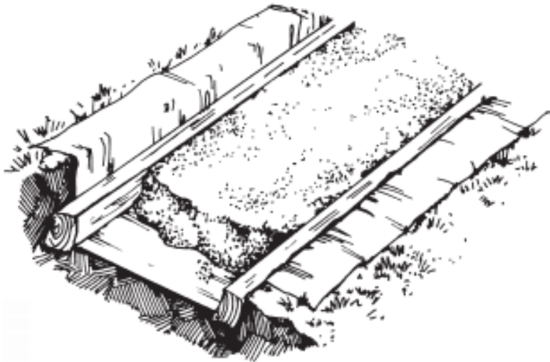
Рис. 21. Устройство подушки
