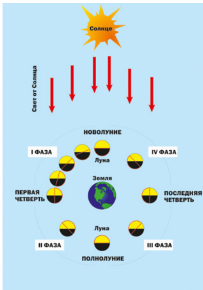
Рис. 9. Вид и порядок смены лунных фаз.
