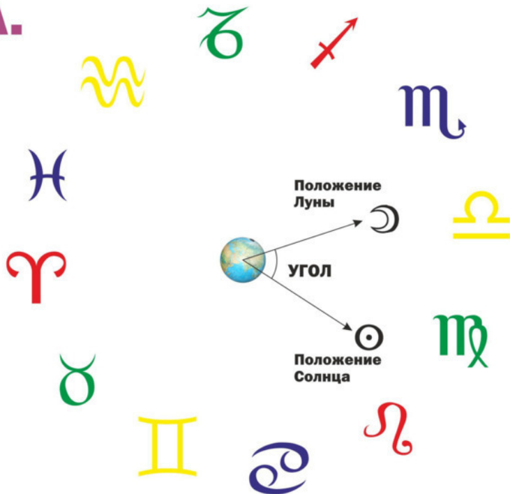
Рис. 8а. Понятие углового расстояния между планетами при наблюдении их с Земли.
