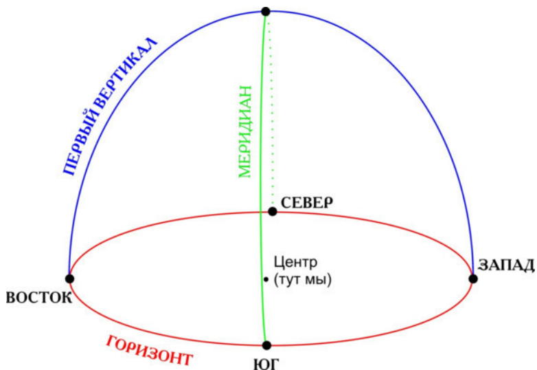
Рис. 11. Расположение 3-х плоскостей пространства.
