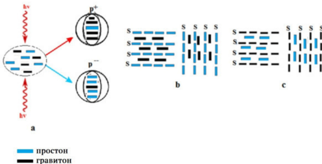
Рис. 2. Схема рождения пары частица – античастица, протон —антипротон, h\nu – фотон, а – рождение пары частица – античастица, б – механизм возникновения массы протона, с – механизм возникновения массы антипротона
