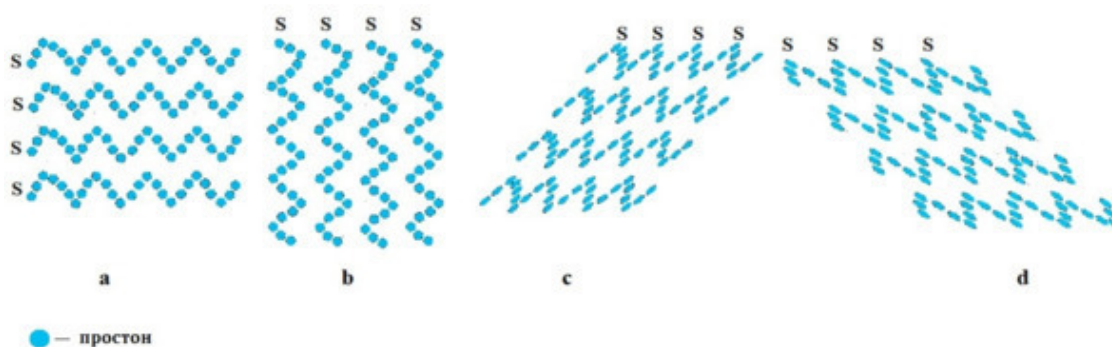
Рис. 1. Предполагаемая схема Мировой сети из силовых нитей пространства, состоящая из простонов.
