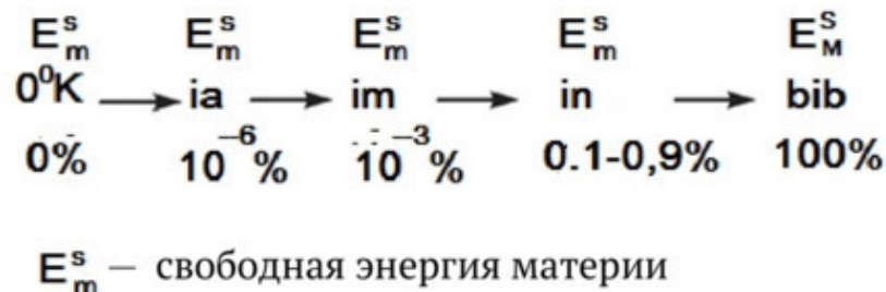
Рис. 4. Соотношение долей свободной энергии к общему объему материальной энергии частицы в зависимости от уровня пространства.
