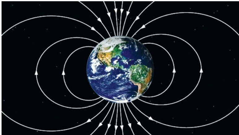
Рис. 2.8. Силовые линии магнитного поля Земли
