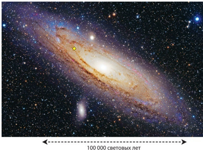
Рис. 2.2. Галактика Андромеды
