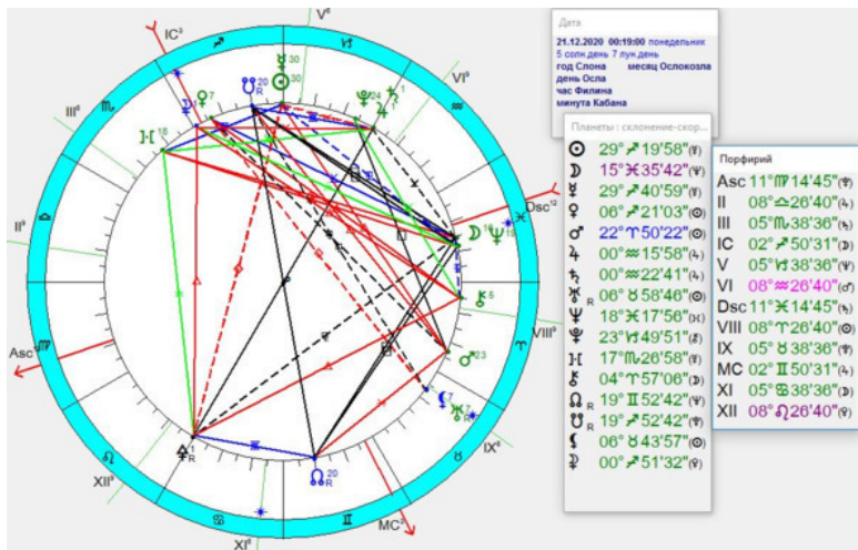
Рис. 4. Супермутация 21.12.2020 г.
