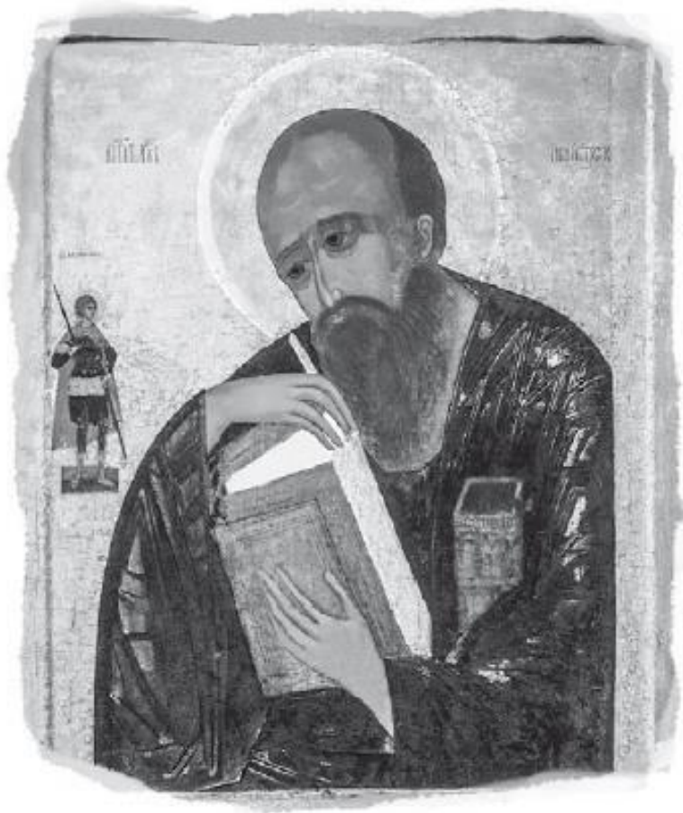
Апостол Иоанн. Икона XVI в
