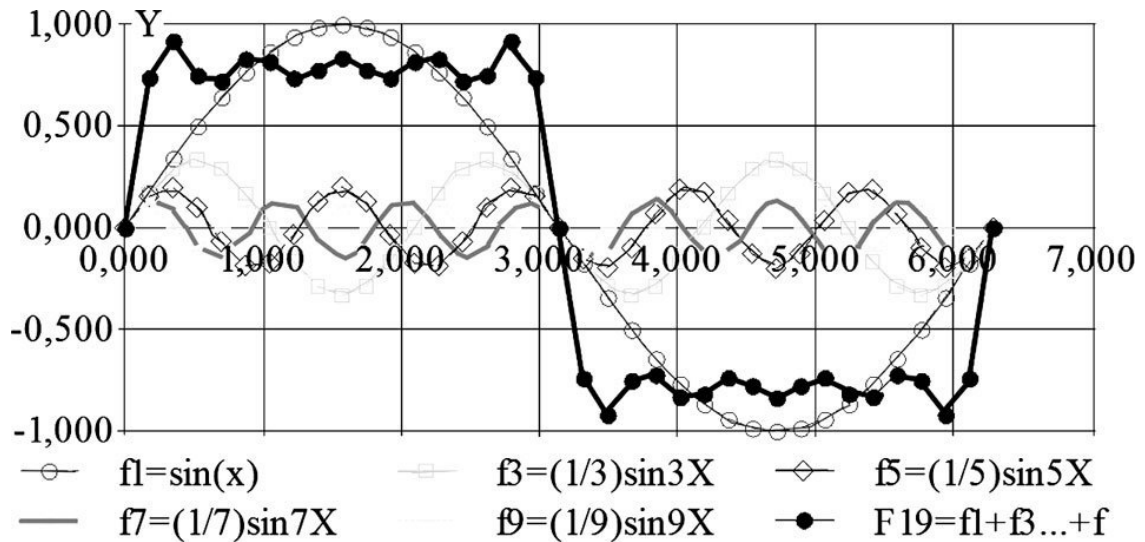
Рис. 1.7. Сложение 1, 3, 5, 7 и 9-й гармоник синусоидального сигнала
