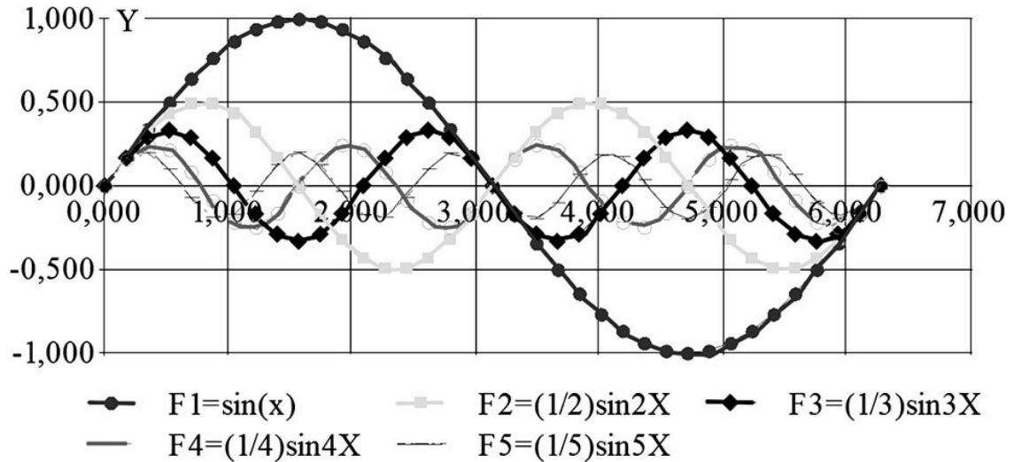
Рис. 1.5. Гармонические составляющие синусоидального сигнала
