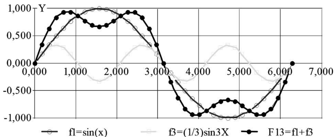
Рис. 1.6. Сложение первой и третьей гармоник синусоидального сигнала
