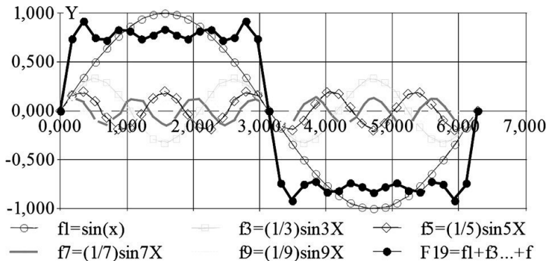
Рис. 1.7. Сложение 1, 3, 5, 7 и 9-й гармоник синусоидального сигнала
