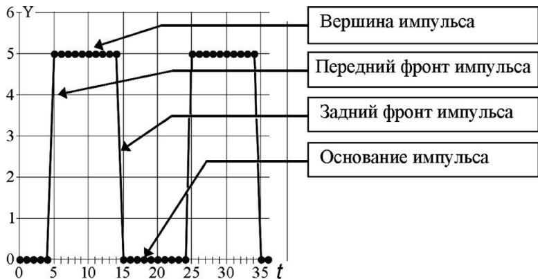
Рис. 1.8. Сигнал импульсной формы
