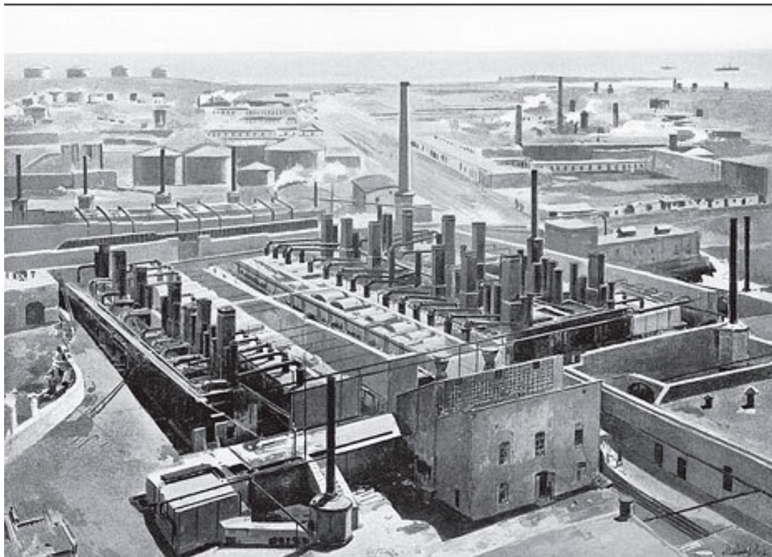
Нефтеперегонный завод Нобелей
