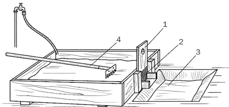
Рис. 9. Гасильный ящик: 1 – задвижка; 2 – сито; 3 – творильная яма; 4 – грабли
