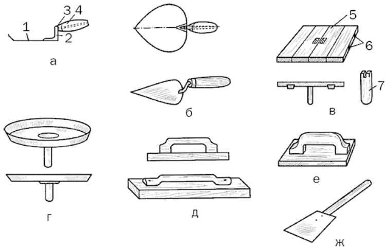
Рис. 4. Инструменты для штукатурных работ: а – штукатурная кельма; б – отрезовка; в – деревянный сокол; г – полутерок; д – терка; е – правило; ж – скребок; 1 – полотно; 2 – колено; 3 – ручка; 4 – черенок; 5 – щит сокола; 6 – шпонки; 7 – ручка сокола
