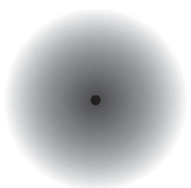
Квантовая волновая функция электрона
