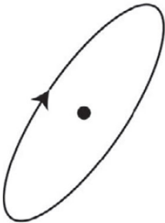
Классическое представление орбиты электрона
