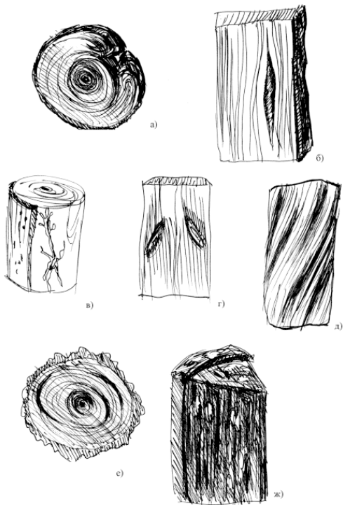
Рис. 2. Пороки строения древесины: а – прорость; б – кармашки; в – чревоотчина; г – сучки; д – косослой; е – свилеватость; ж – гнили
