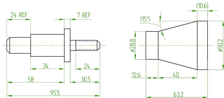
Рисунок 12 – Обозначение справочных размеров
