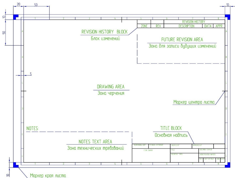
Рисунок 1 – Структура чертежного листа
