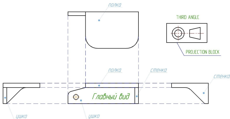
Рисунок 4 – Иллюстрация расположения видов по методу первого угла
