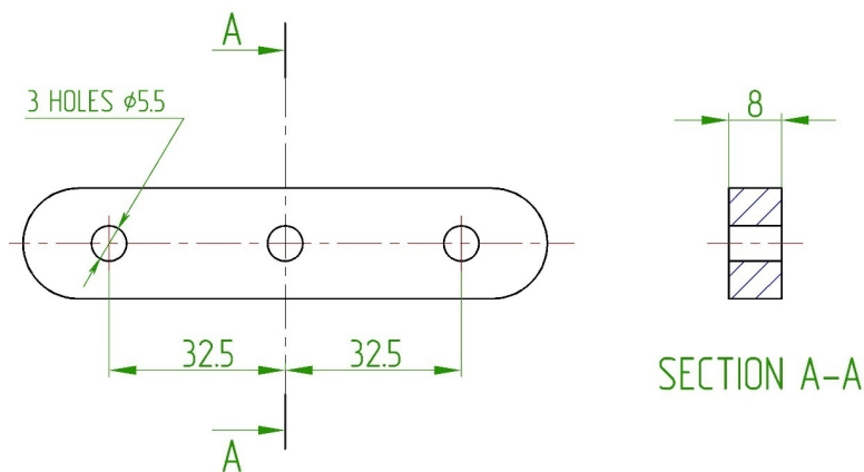
Рисунок 16 – Размеры отверстий
