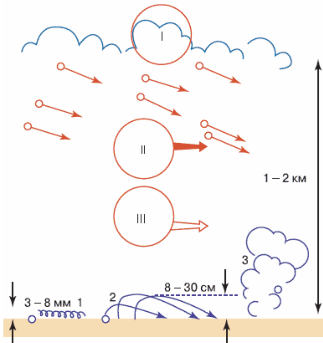
Движение снега во время метели: I – верховая метель; II – общая метель; III – низовая метель (1 – влечение снежинок, 2 – сальтация снежинок, 3 – диффузия снега)
