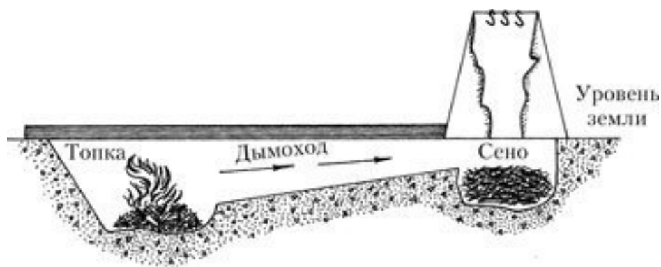
Рис. 10. Траншея-коптильня на территории дачного участка
