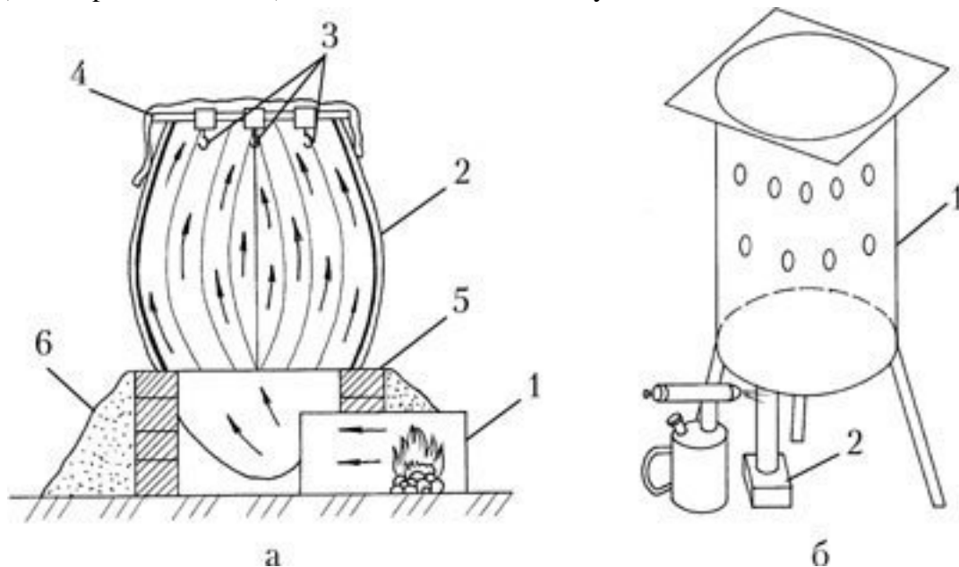
Рис. 24. Варианты коптилен из бочек:
