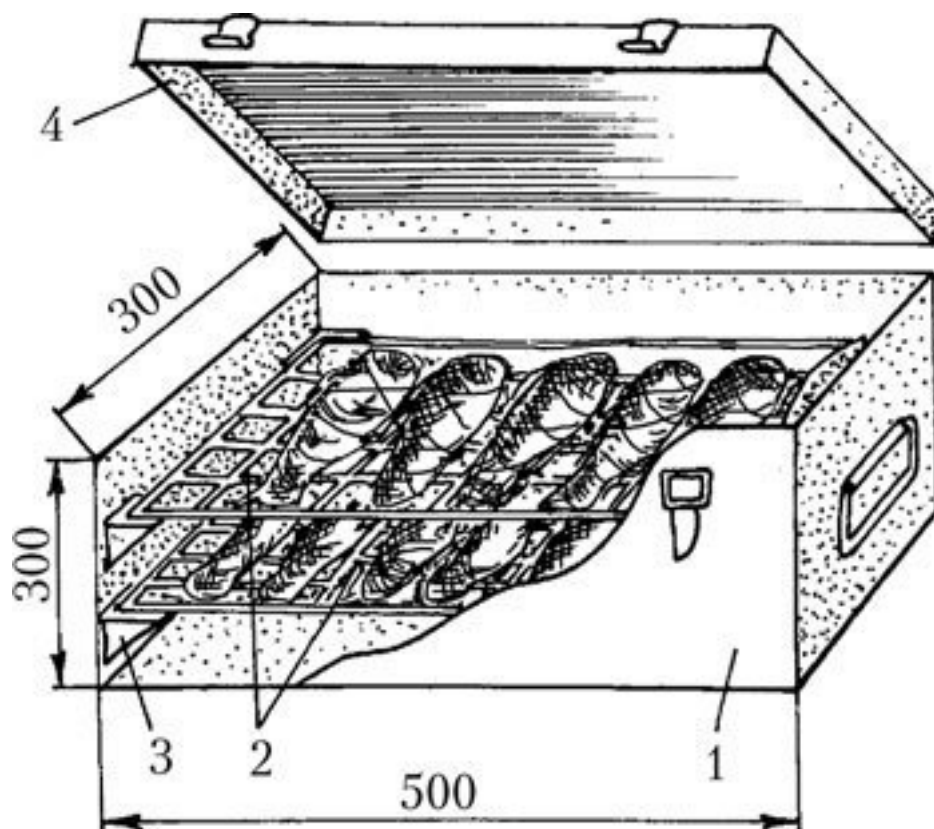
Рис. 7. Переносная коптильня в виде ящика:
