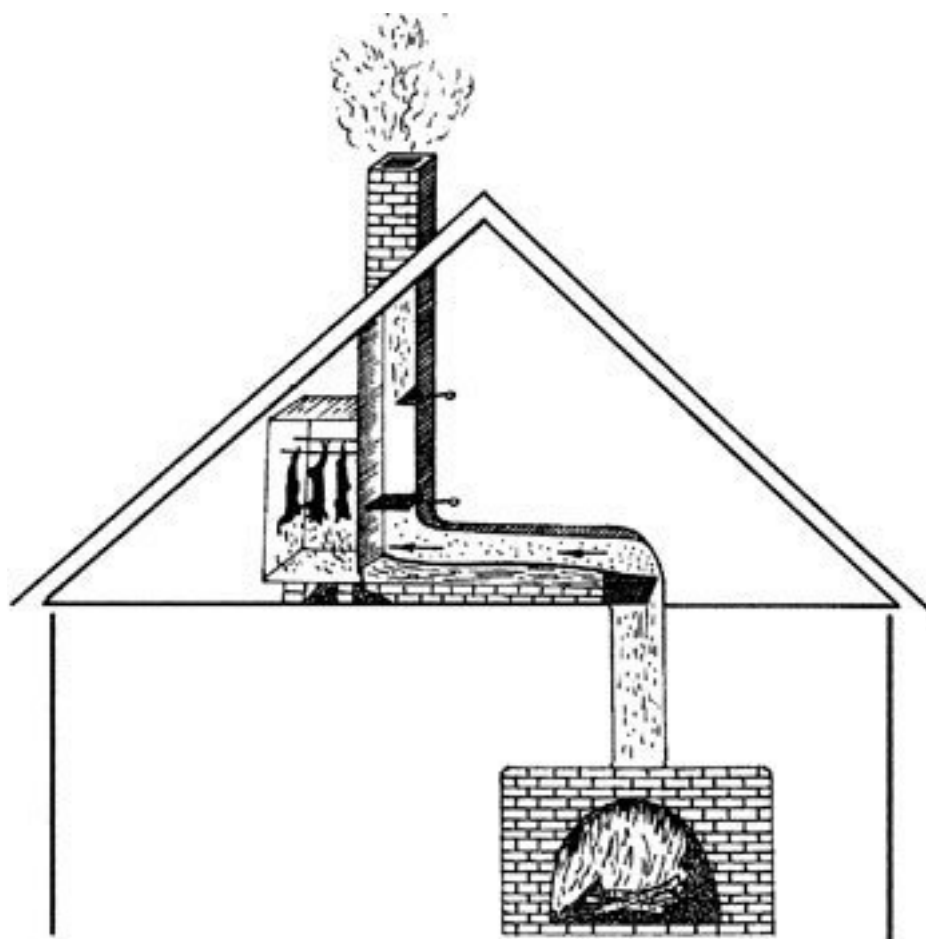
Рис. 9. Домашняя коптильня на чердаке
