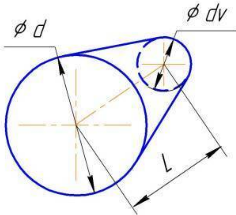
Рис. Конус усеченный.
