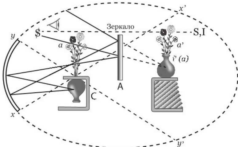
Рисунок 2. Конструкция с двумя зеркалами
