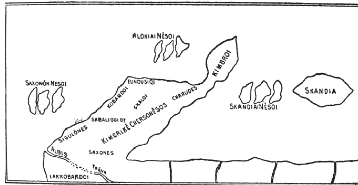
Рис. 1 Север Птолемея
