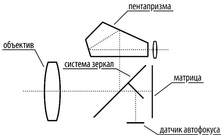
Схема 1. Устройство зеркальной камеры.
