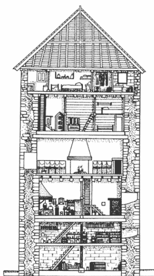
Разрез жилой башни, типичной для раннесредневековой Германии
