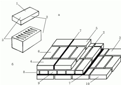
Рис. 21. а – стороны кирпича и камня; б – элементы ка-менной кладки: 1 – постель; 2 – ложок; 3 – тычок; 4 – наруж-
