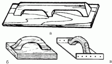
Рис. 12. Инструменты для оштукатуривания: а – полуте-
