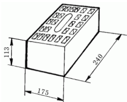
Рис. 20. Массивный кирпич (размеры даны в мм).
