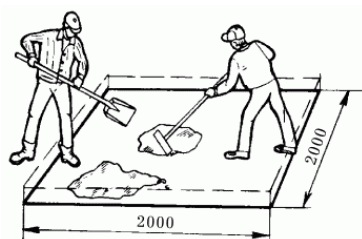
Рис. 15. Площадка для замеса растворов (размеры даны
