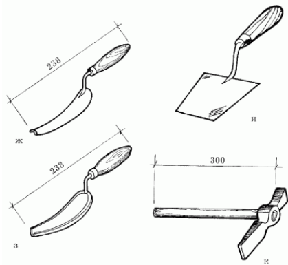
Рис. 11 (продолжение). Инструменты для кладки кирпича и оштукатуривания (размеры даны в мм): ж, з – расшивки; и – кельма; к – молоток-кирочка.
