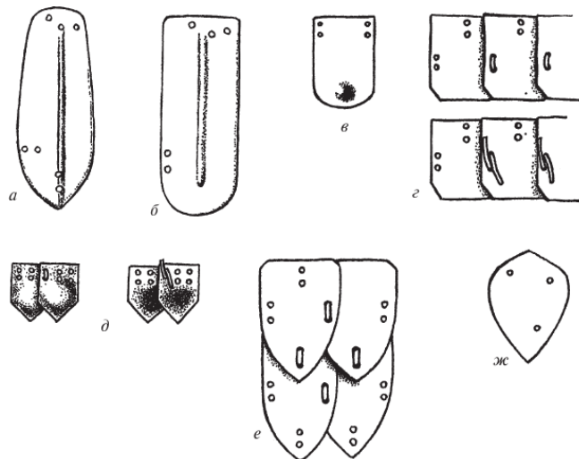
Рис. 2. Разновидности пластин для доспехов: а – египетская, бронза, XVII в. до н. э. (музей Метрополитен, Нью-Йорк); б – сирийская, из Низы, XV в. до н. э. (Багдадский музей); в – египетская с выступом, из гробницы фараона, X в. до н. э. (Бруклинский музей); г – римская, бронза, из Авентикума (Земельный музей, Цюрих); д – римская, бронза, по Корбриджу (министерство общественных построек и работ, Лондон); е – римская, бронза, из Сотина (Загребский музей); ж – китайская, медь, из Синганя, династия Хань, по Лауферу
