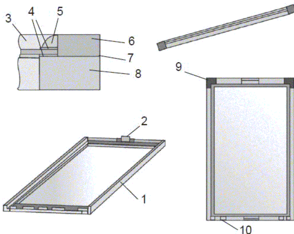
Рис. 8. Изготовление парниковых рам: 1 — рама по размеру стекла; 2 — ручка; 3 — стекло; 4 — замазка с двух сторон; 5 — штапик или гвозди с замазкой; 6 — брусок 40×20 мм; 7 — место склейки водоустойчивым клеем; 8 — брусок 55×30 мм; 9 — стальной угольник; 10 — накладка для упора.
