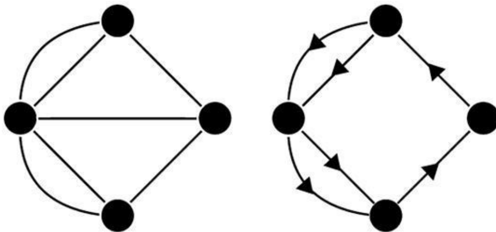
Илл. 5. Упрощенная схема Эйлеровой задачи о кёнигсбергских мостах. Задачу можно решить, только убрав грань в середине (то есть мост, соединяющий два острова, на илл. 4).
