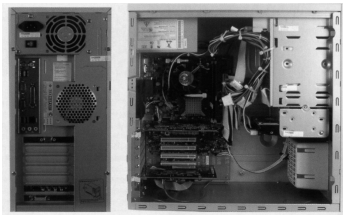
Системный блок
