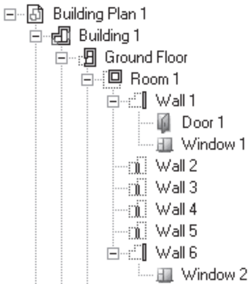
Рис. 1.1. Пример иерархического представления строительного плана, созданного на основе объектного подхода
