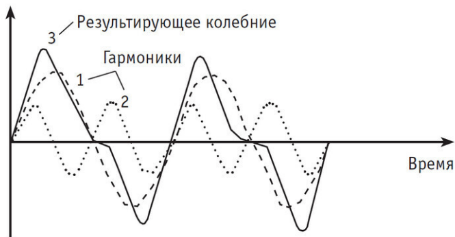
Рис. 3. Пример разложения периодического колебания (кривая 3) на гармоники (кривые 1 и 2)
