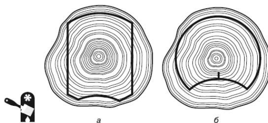
Рис. 1.9. Профилирование бруса (а) и оцилиндровка бревна (б)
