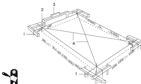
Рис. 2.1. Разметка площадки под фундамент: 1 – обноска из досок; 2 – отвес; 3 – уровень; 4 – шнур
