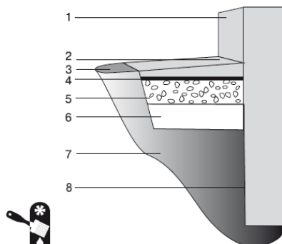
Рис. 2.6. Схема отмостки без утепления: 1 – цоколь; 2 – бетонное покрытие; 3 – растительный слой; 4 – арматурная сетка; 5 – слой щебня; 6 – слой песка; 7 – грунт; 8 – фундамент
