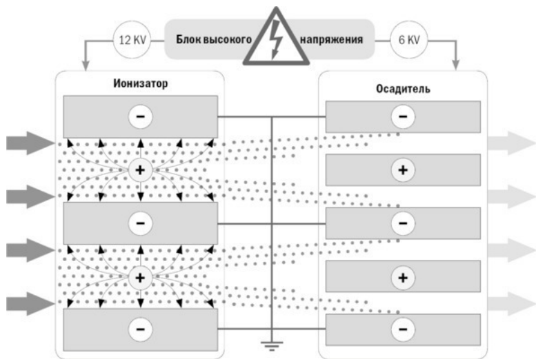
Рисунок 44. Электростатический фильтр для улавливания аэрозолей
