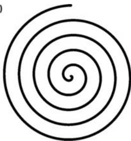
Рисунок 25. Спираль Архимеда: а – правая (вращение против часовой стрелки); б – левая (вращение по часовой стрелке)
