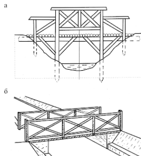
Рис. 1. Типы простейших конструкций мостиков
