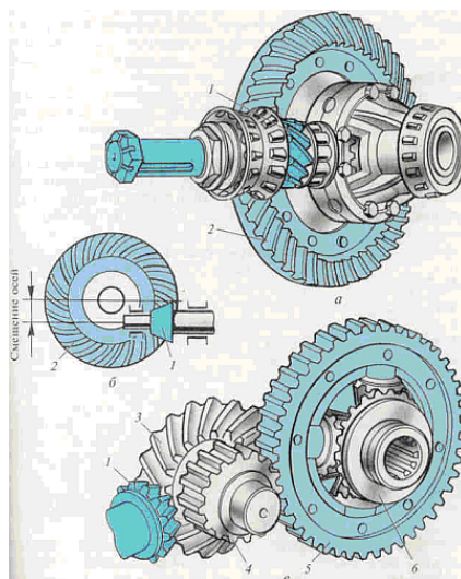
Рис. Главная передача. А – обычная передача, б – одинарная гипоидная. В – двойная, 1 – ведущая шестерня с валом, 2 – ведомая коническая шестерня, 3 – промежуточная шестерня, 4 – промежуточная цилиндрическая шестерня с валом, 5 – ведомая цилиндрическая шестерня, 6 – дифференциал.
